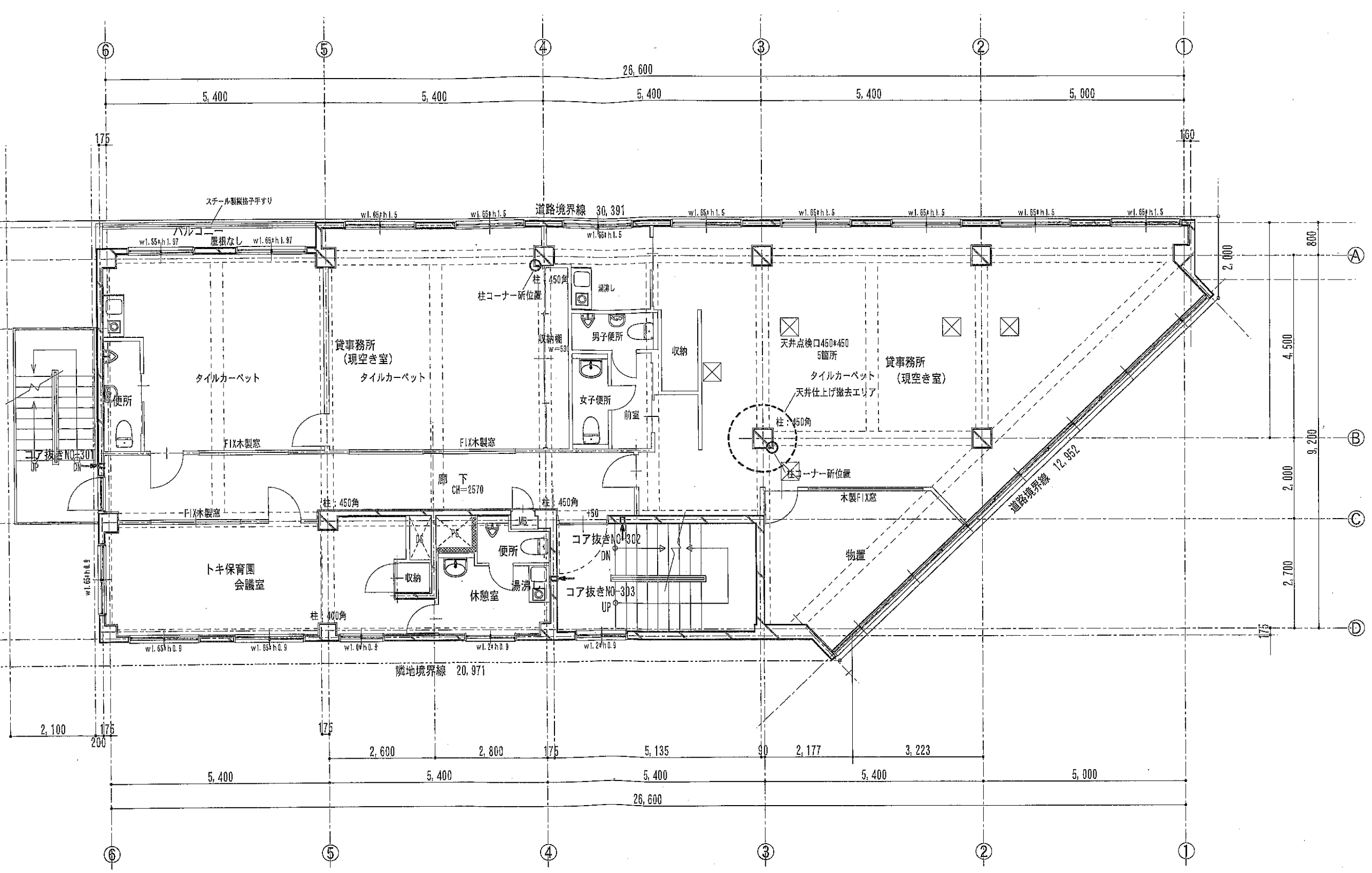
2階 平面図 1/200
